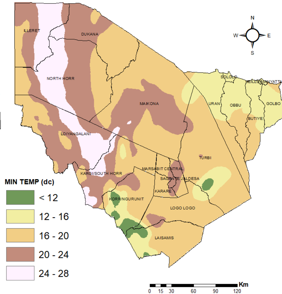
7 WEEKLY MINIMUM TEMP FST VALID 3 - 9 FEB 2026
